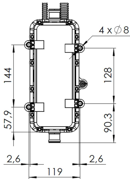
Rysunek 1 Wymiary otworów montażowych – grzałka cieczy PTC
